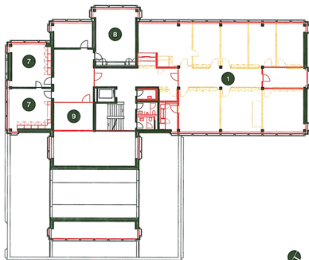
2. Obergeschoss
